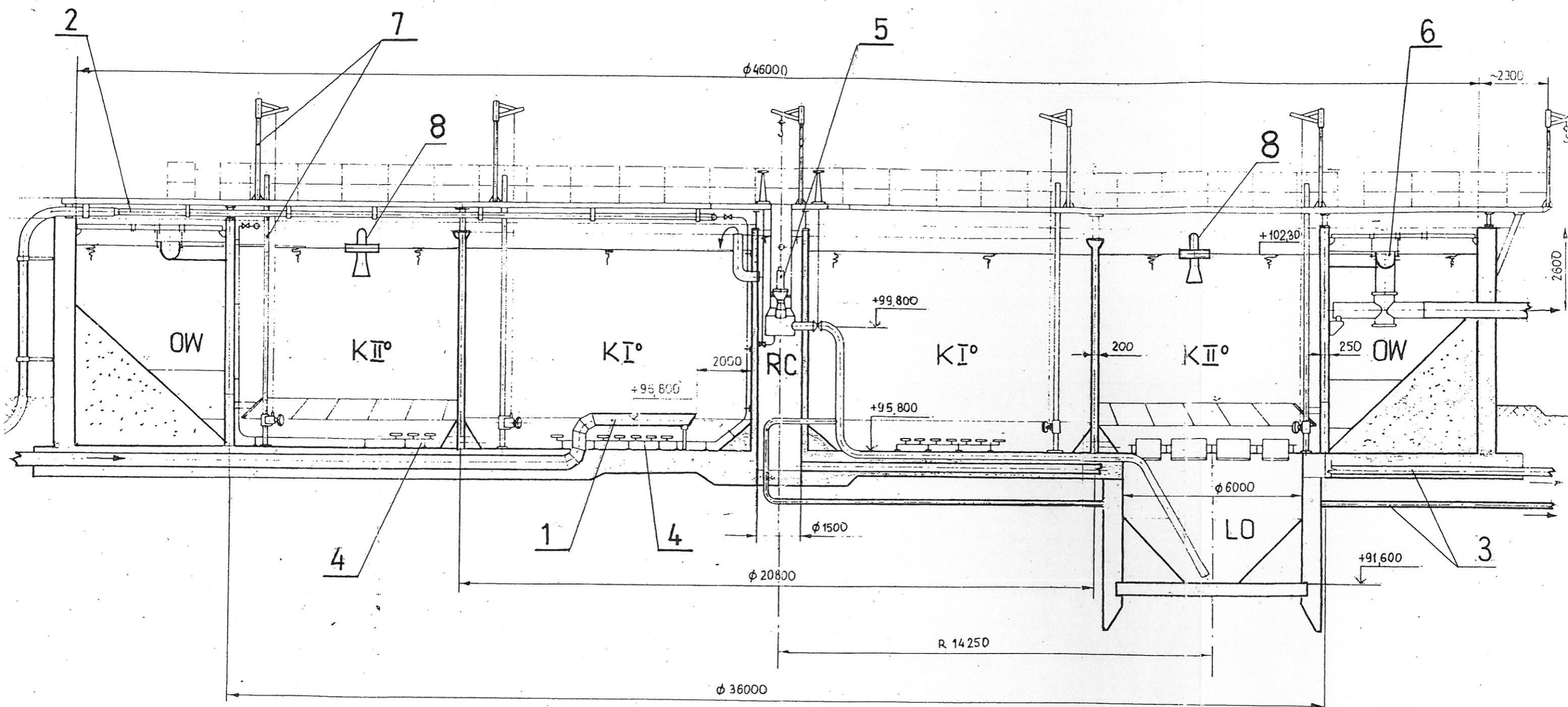
Rys. 5. Przekrój reaktora BIOMIX przeznaczonego na zbiornik retencyjny.
