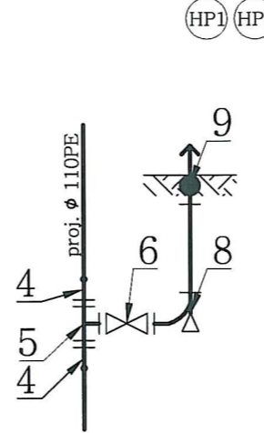
Węzeł hydrantu HP1 HP2
