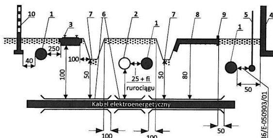
TABLICA ODLEGŁOŚCI KABLI ELEKTROENERGETYCZNYCH I SYGNALIZACYJNYCH UŁOŻONYCH BEZPOŚREDNIO W ZIEMI DO INNYCH URZĄDZEŃ PODZIEMNYCH wg N SEP-E-004
